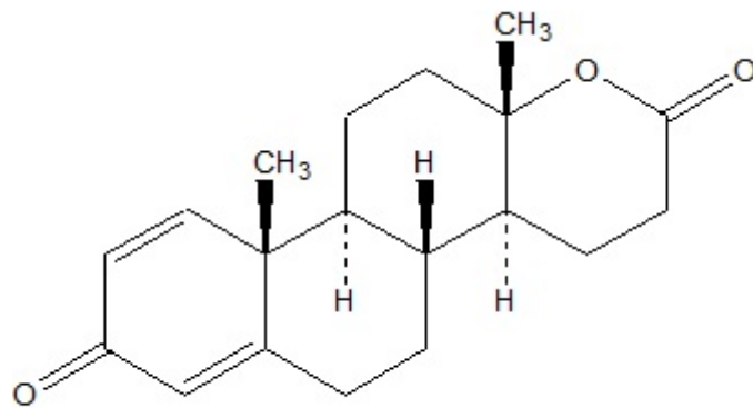
Testolactone
